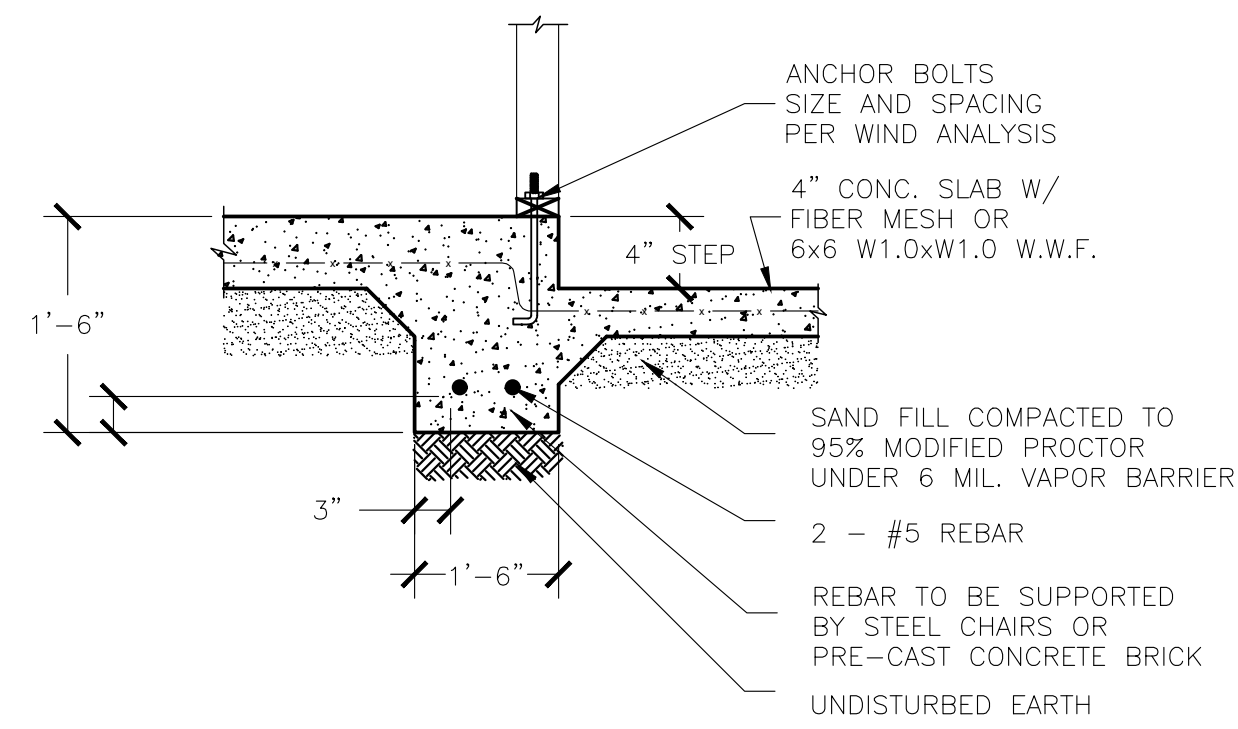
E STEPDOWN DETAIL SCALE: 3/4"=1'-0"
